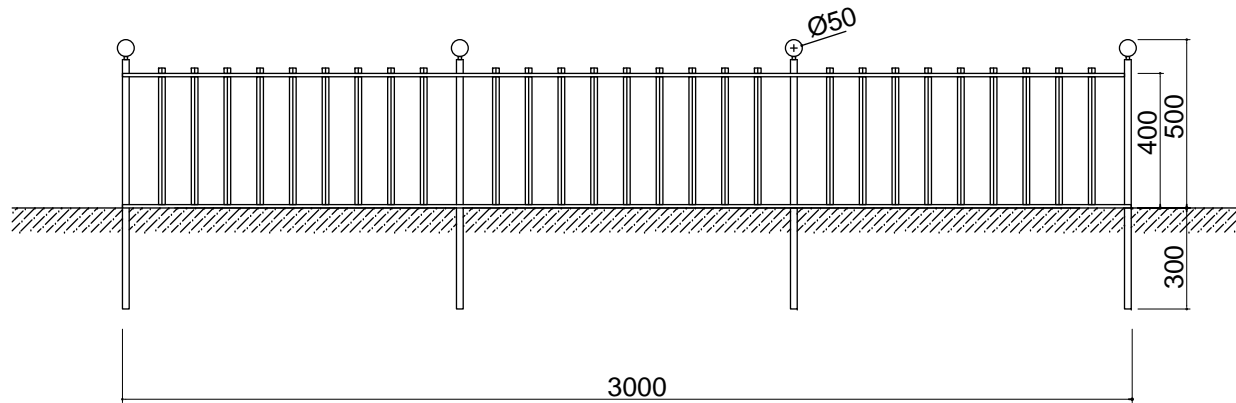
ALZADO FRONTAL
