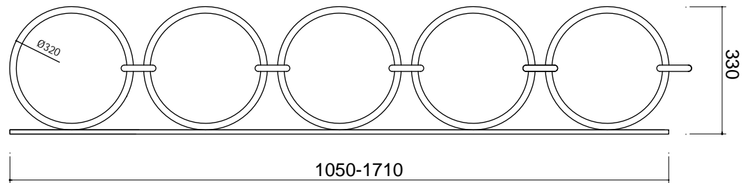
ALZADO
