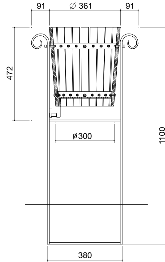
SECCION
