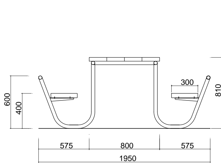
SECCIÓN
